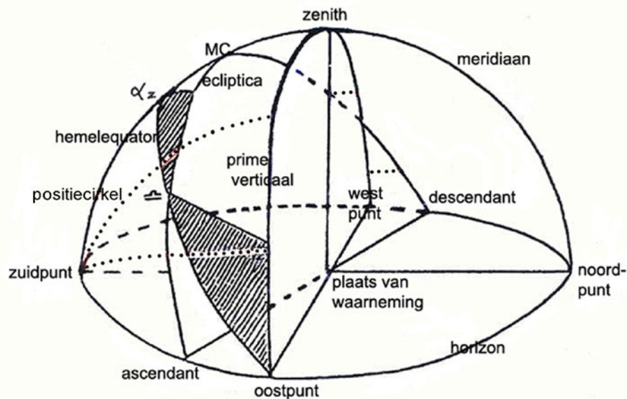
Positieciikels (stippellijn) brengen de planeten en sectorgrenzen over op de Prime Verticaal
